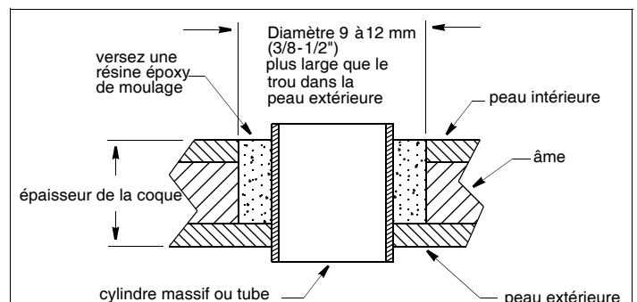
Figure 4. Préparation d'une coque en sandwich
