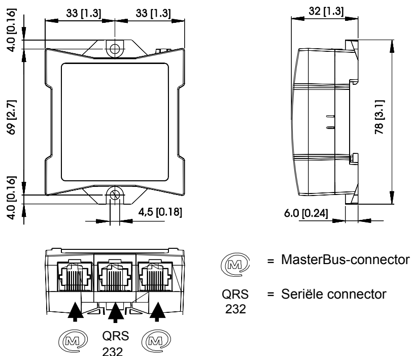
Afbeelding 2: Afmetingen in mm [inches] en connectoren
