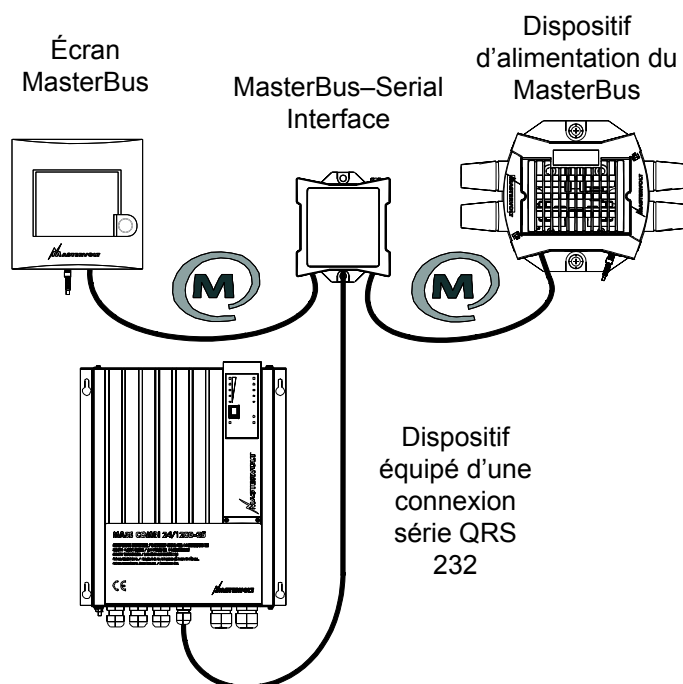
Figure 1 : MasterBus–Interface série intégrée
