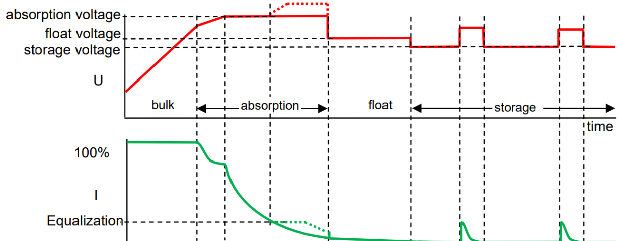
Illustration 3 Tension et courant durant les différents états de charge de la batterie
