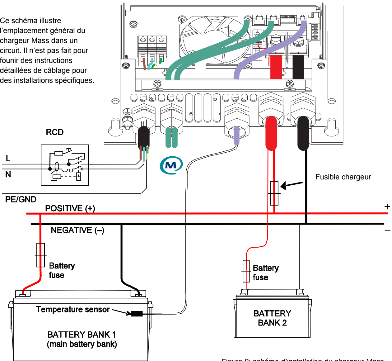
Figure 8: schéma d'installation du chargeur Mass
