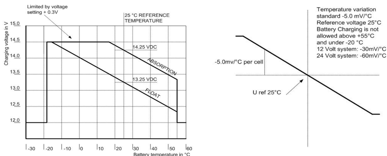
Figure 17: Caractéristique de la compensation de température (tension de charge versus température)
