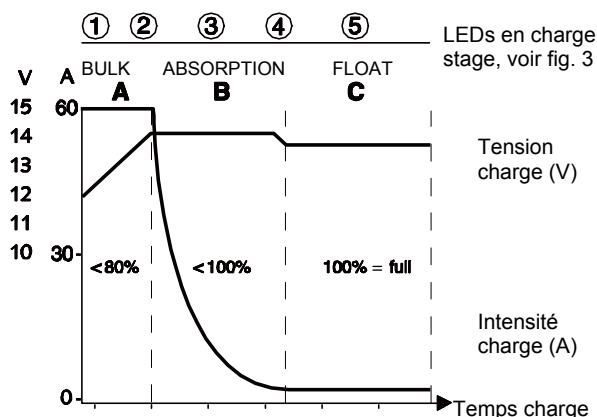
Fig. 2 : Exemple : caractéristique de charge du MASS 12/60-2. (Pour les autres modèles, V/A [tension et intensité] selon les fiches techniques.)
