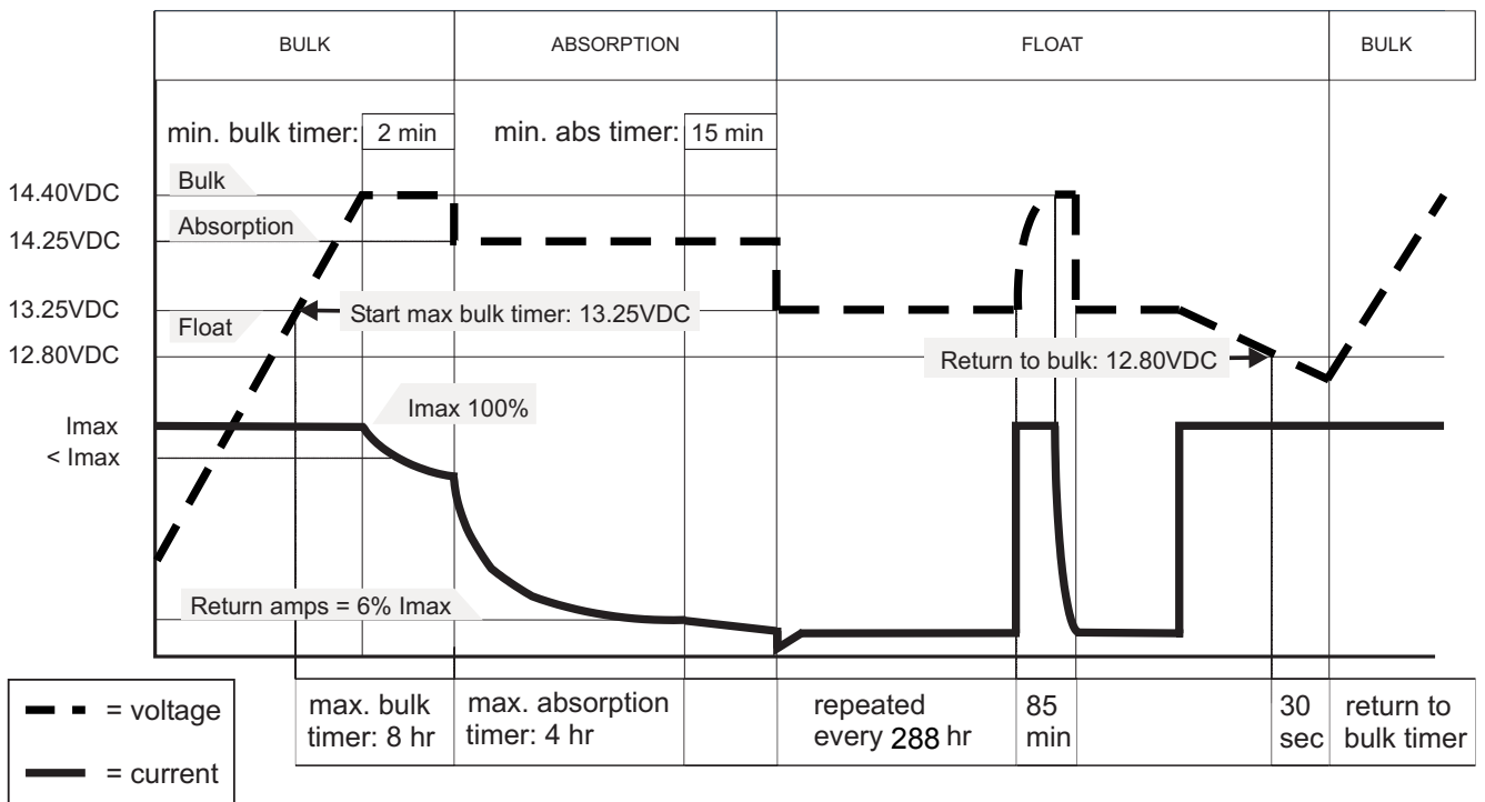
Figure 10 : caractéristiques de charge de la méthode de charge à trois étapes Plus (@ 25°C / 77°F)
